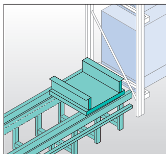
チェーンコンベヤ
